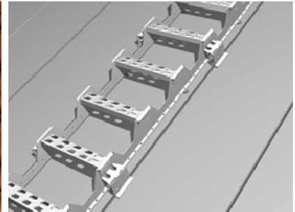
Kuva 3. Saumapelti- ja Classic-katto
