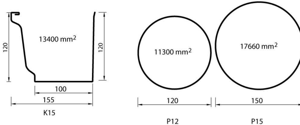
Kuva 1. Läpileikkauspinta-alat
