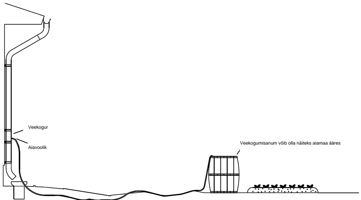
Joonis 2. Veekoguri tööpõhimõte
