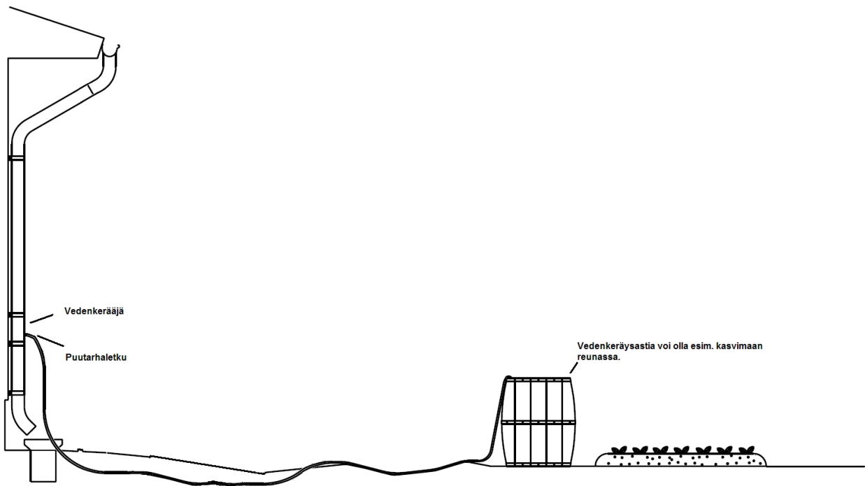
Bild 2. Vattenuppsamlarens funktionsprincip
