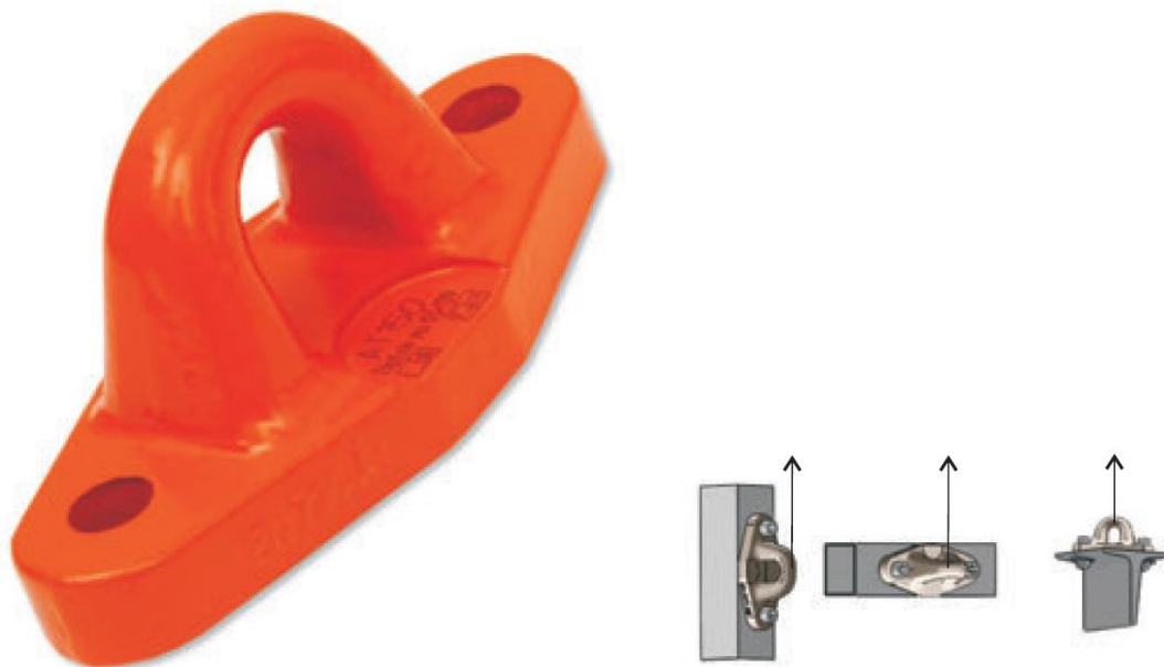
Bild 1. Fästpunkter och godkända användningsriktningar
